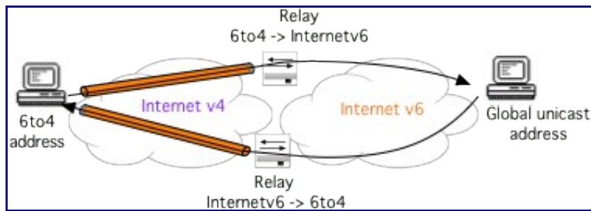
Figure 9: Routage asymétrique.
