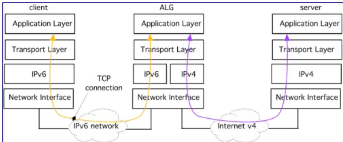
Figure 1: Communication par passerelle applicative.
