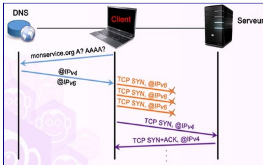
Figure 5: Etablissement de connexion d'un client en double pile.
