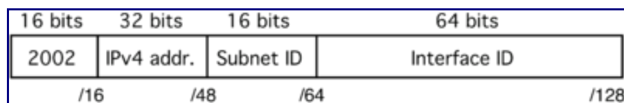
Figure 6: Format d'une adresse 6to4.
