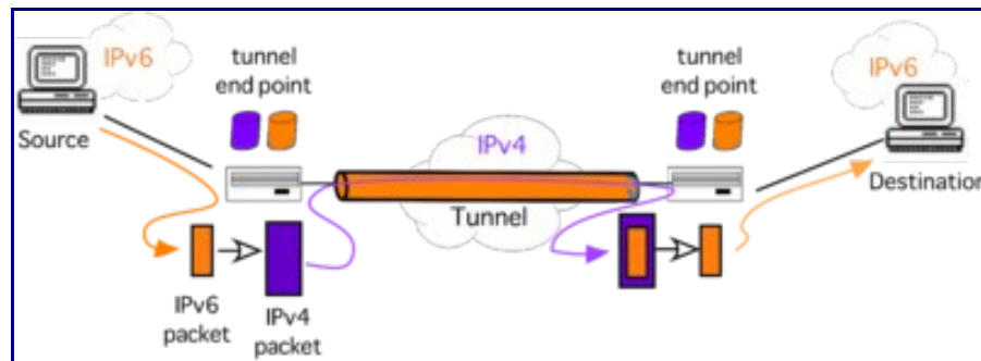
Figure 2: Tunnel entre des réseaux IPv6.
