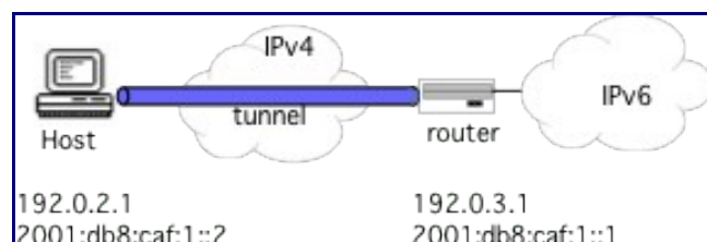
Figure 4: Cas d'un tunnel configuré.
