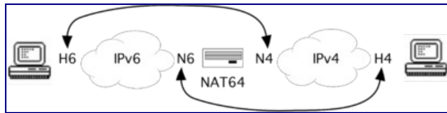
Figure 2: Les adresses utilisées pour la traduction.
