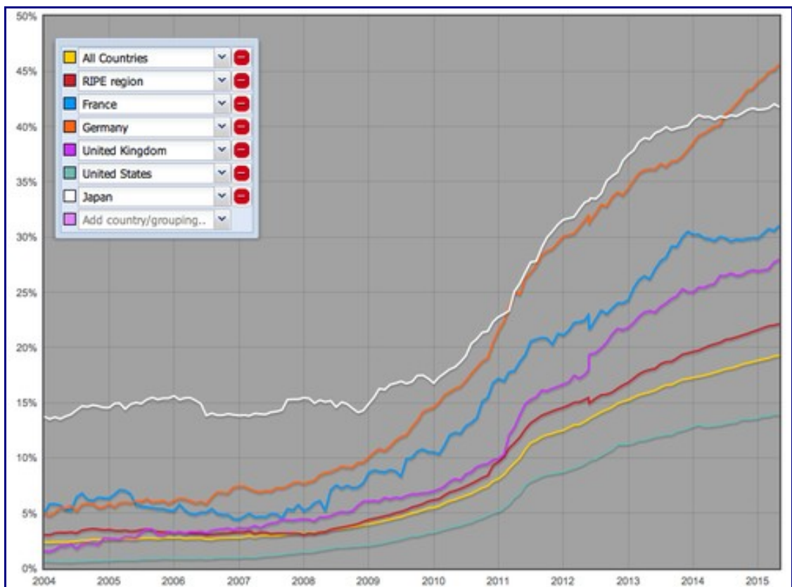
Figure 4: Evolution du pourcentage d'organisations annonçant au moins un préfixe IPv6 par région.
