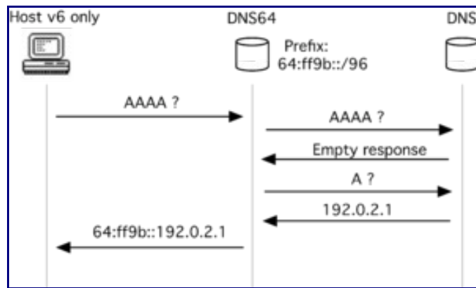
Figure 3: Opérations du DNS64.
