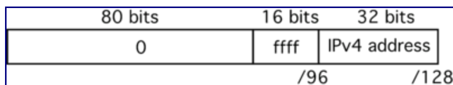
Figure 4: Adresse IPv4 imbriquée dans une adresse IPv6.
