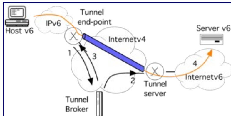
Figure 11: Configuration d'un Tunnel Broker avec TSP.
