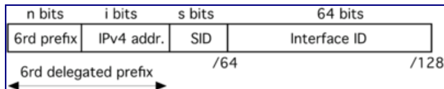
Figure 13: Format d'une adresse 6rd.
