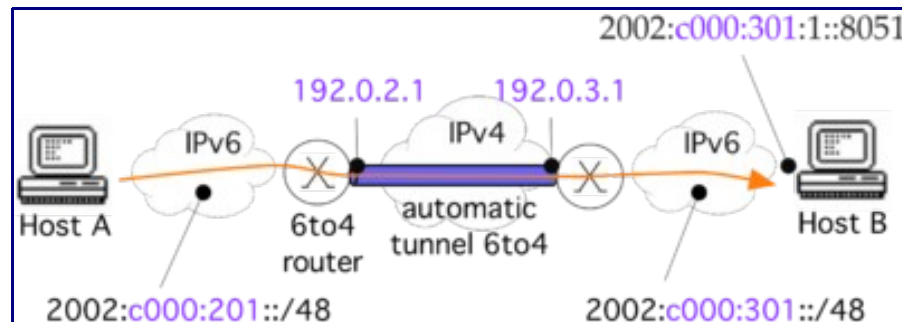
Figure 8: Acheminement d'un paquet IPv6 en 6to4.
