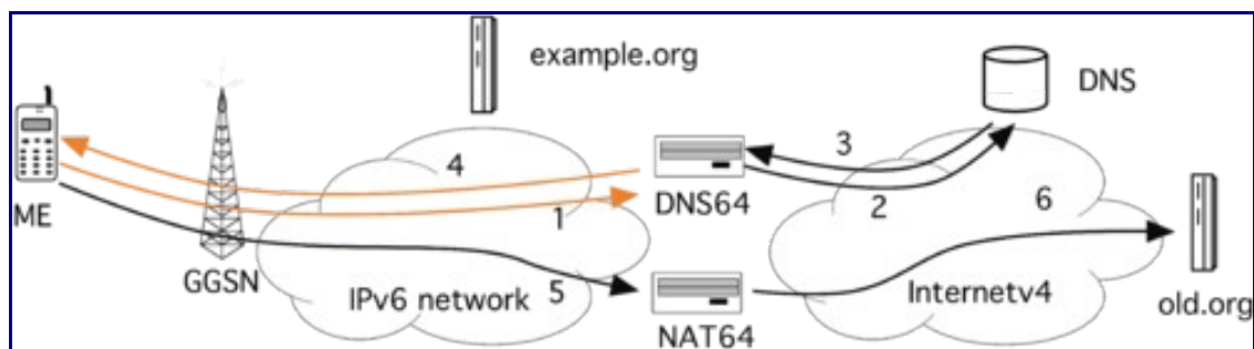
Figure 7: Accès à un serveur en IPv4.
