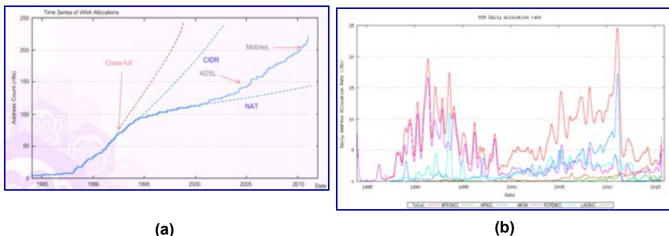
Figure 1: Cumul de consommation des adresses IPv4 et taux de consommation.
